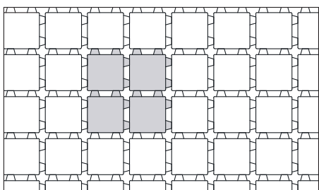
název KARO EKO orientační ukázka POMĚR BETON/ OTVOR beton 80,5 % otvor 19,5 %
