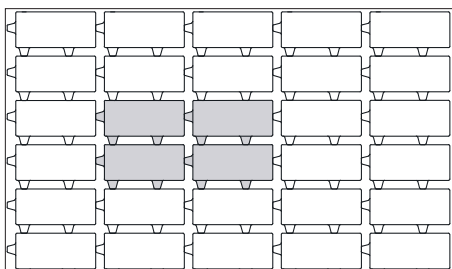
název PALLADIO EKO II orientační ukázka POMĚR BETON/ OTVOR beton 77,7 % otvor 22,3 %
