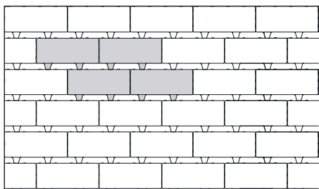
název PALLADIO EKO I orientační ukázka POMĚR BETON/ OTVOR beton 84,7 % otvor 15,3 %
